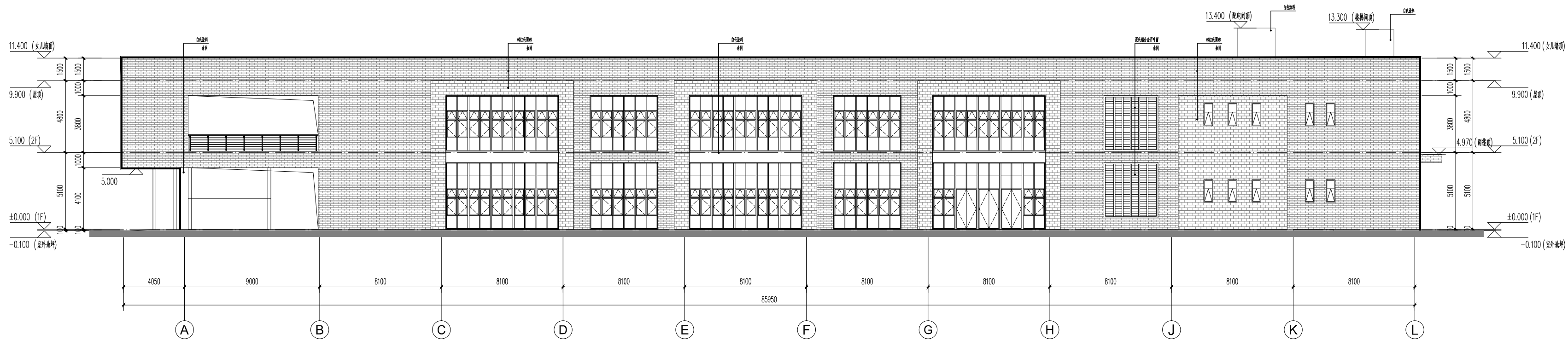
东立面 1:150
