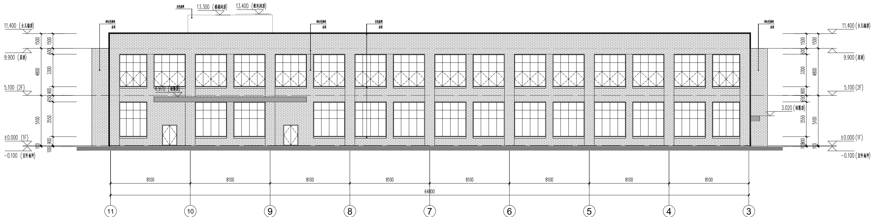
北立面 1:150
