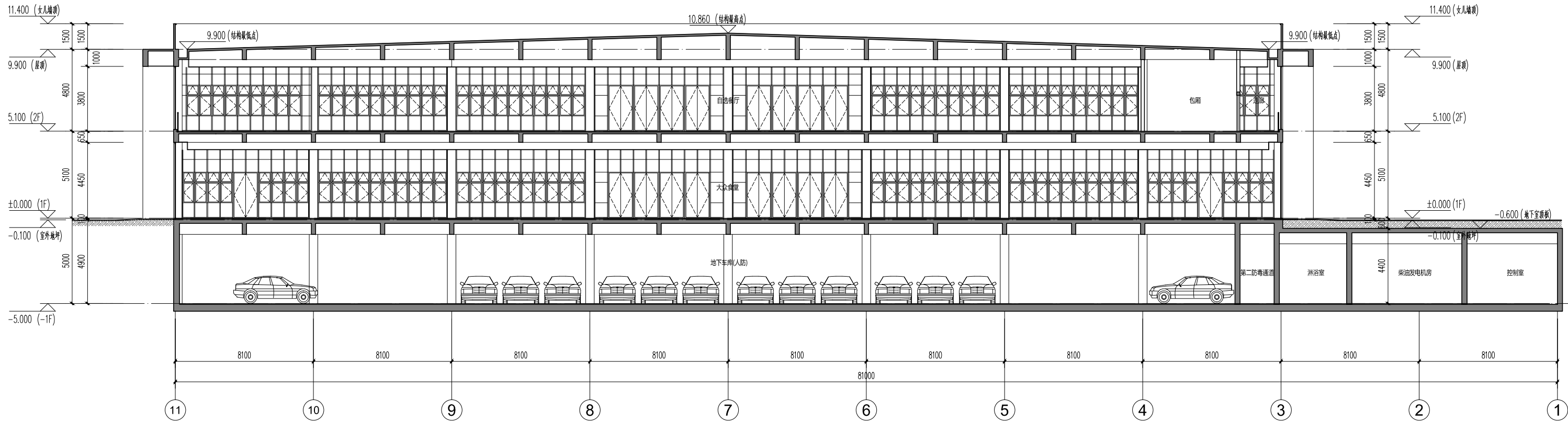
2-2剖面图 1:150
