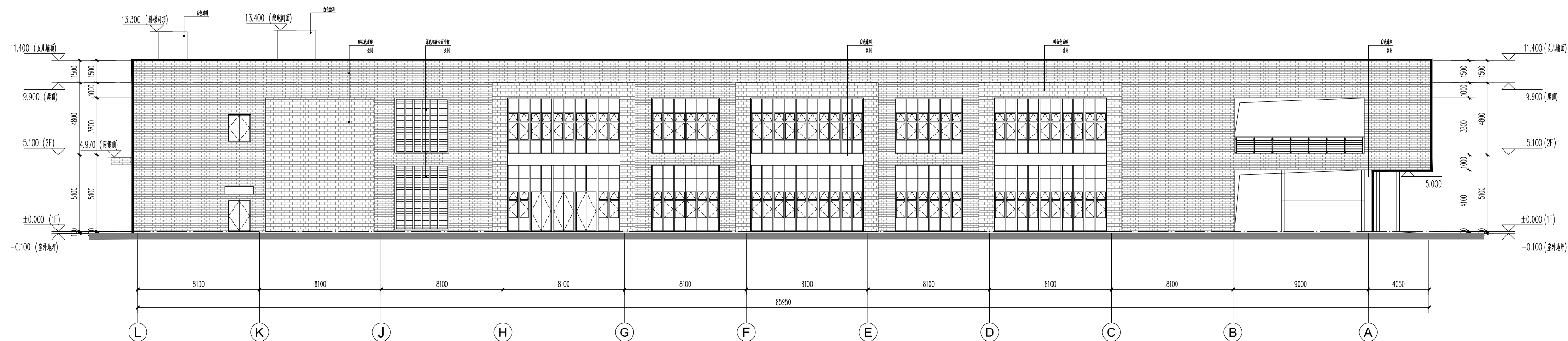
西立面 1:150
