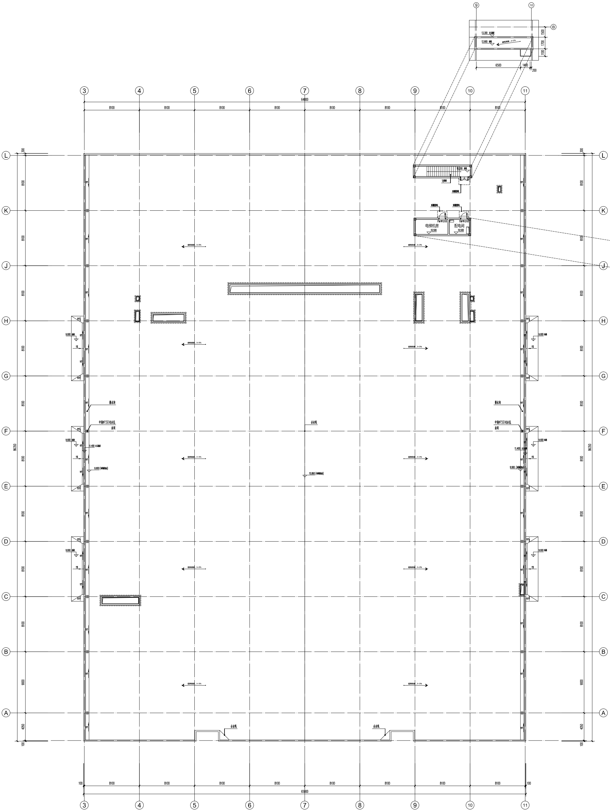
屋顶平面图 1:150 注:10表示雨水口,11表示雨水管。
